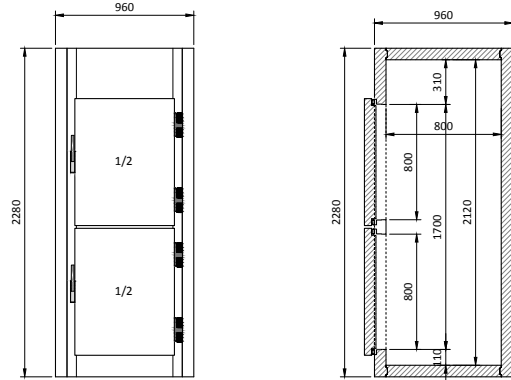
Hauteur 2280 mm
