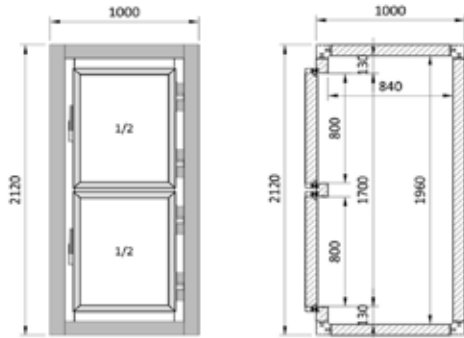
Hauteur 2120 mm
