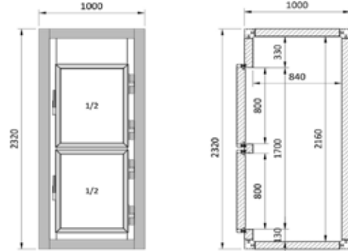
Hauteur 2320 mm
